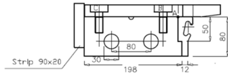
Figuur 1 Standaard ESCOjoint 60s
